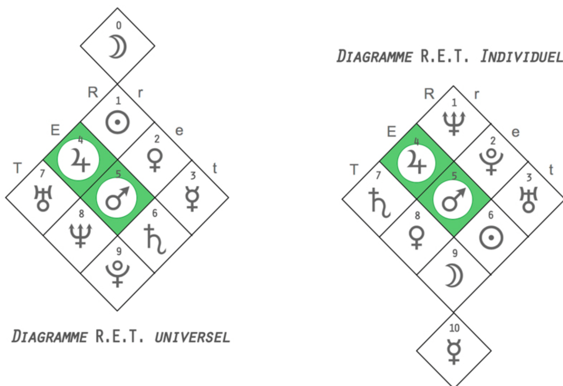
Fig 2 : La comparaison du Diagramme R.E.T. universel et du diagramme R.E.T. individuel permet de définir le ou les domiciles planétaires. Ici, Mars et Jupiter (4 e et 5 e rangs de la hiérarchie individuelle des puissances planétaires) sont à leur place naturelle puisque ces deux planètes occupent le même rang qu'elles ont et qui est leur lieu naturel dans la hiérarchie universelle.
