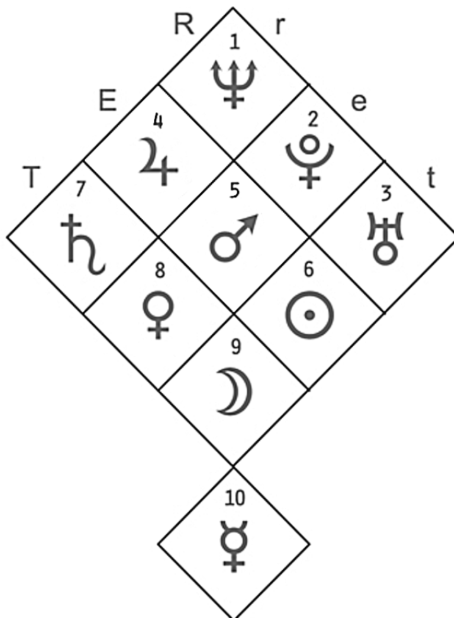
Fig 1 : la hiérarchie des puissances planétaires peut être représentée de la sorte dans le diagramme R.E.T.
